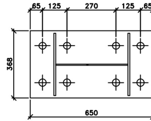
BASE PLATE D2A & D2B
