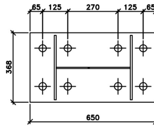
BASE PLATE D2A & D2B
